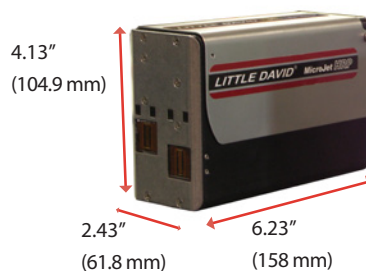
MicroJet HRP 1"
