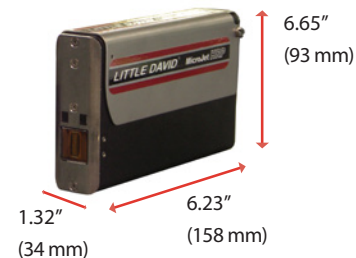
MicroJet HRP 1/2"
